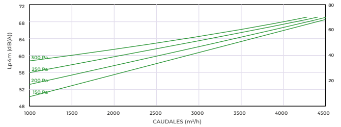
SIBERDUO RM 9035
