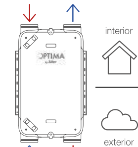
Modelo flujos de aire versión izquierda Ref: DFOPTIMA1BPL
