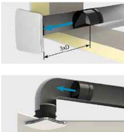
FLOW con regulador MRR en insuflación
