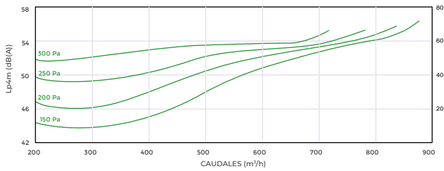
SIBERDUO RM 9010
