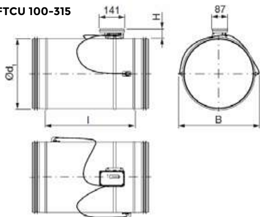
FTCU 100-315
