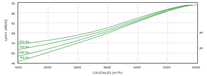
SIBERDUO RM 9048
