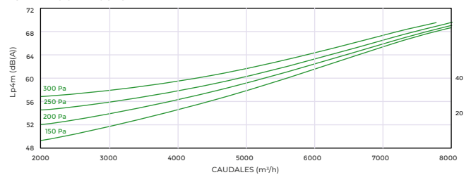
SIBERDUO RM 9070
